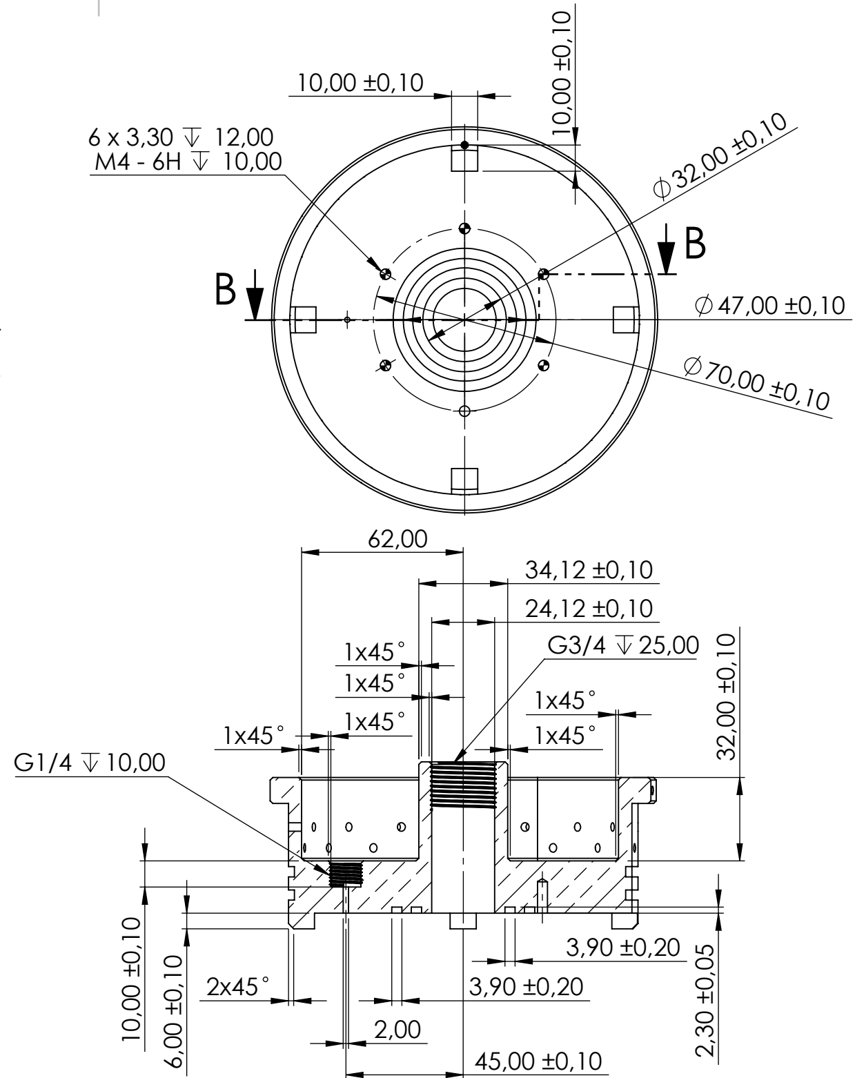
PRZEKRÓJ B-B
